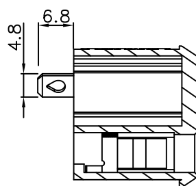
截面:A-A
